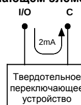
Выход управления на твердотельном переключающем элементе
